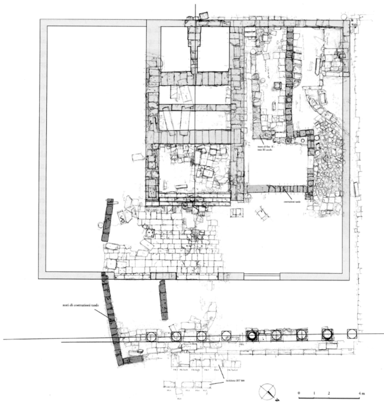
Fig. 5 – Leptis Magna, tempio della Magna Mater. Pianta del santuario. Rilievo e disegno dell'autore.
