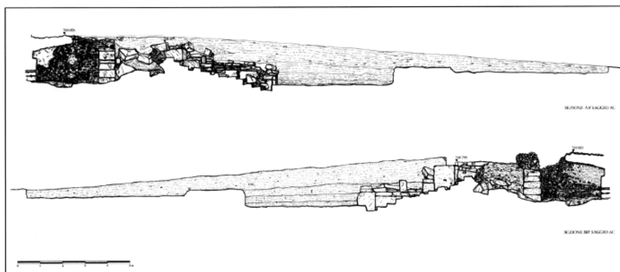
Fig. 11 – Althiburos, teatro. Sezioni lungo l'asse dell'edificio, Saggio A, 2009. Rilievo di Antonello Fino, Fernando Giannella, Luca Schepisi, disegno di Paola Pietanza, Valentina Santoro, Antonello Fino (Politecnico di Bari).
